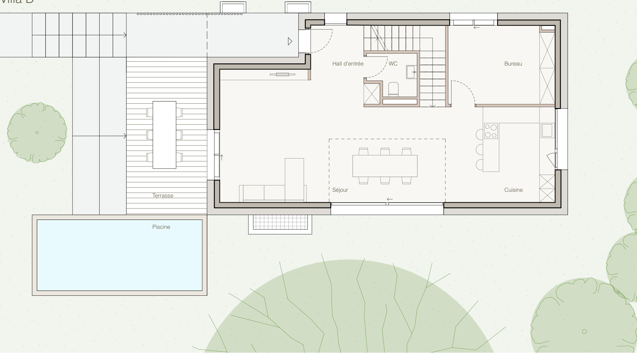
PLAN REZ-DE-CHAUSSEE Surface rez-de-chaussée: 71 m²
